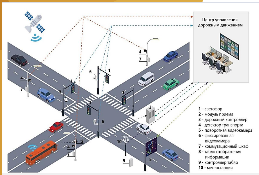
Схема организации автоматизированной системы управления дорожным движением «Зеленая волна»
